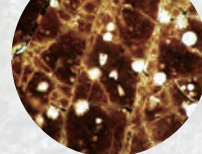
プランクトンの化石を含む赤色チャート ＜南アルプス(中央構造線エリア)ジオパーク/長野県＞
