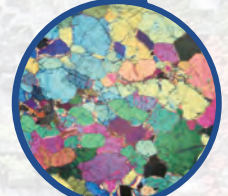
地球深部で生まれたかんらん岩とその偏光顕微鏡写真 ★ ＜アホイ岳ユネスコ世界ジオパーク/北海道＞
